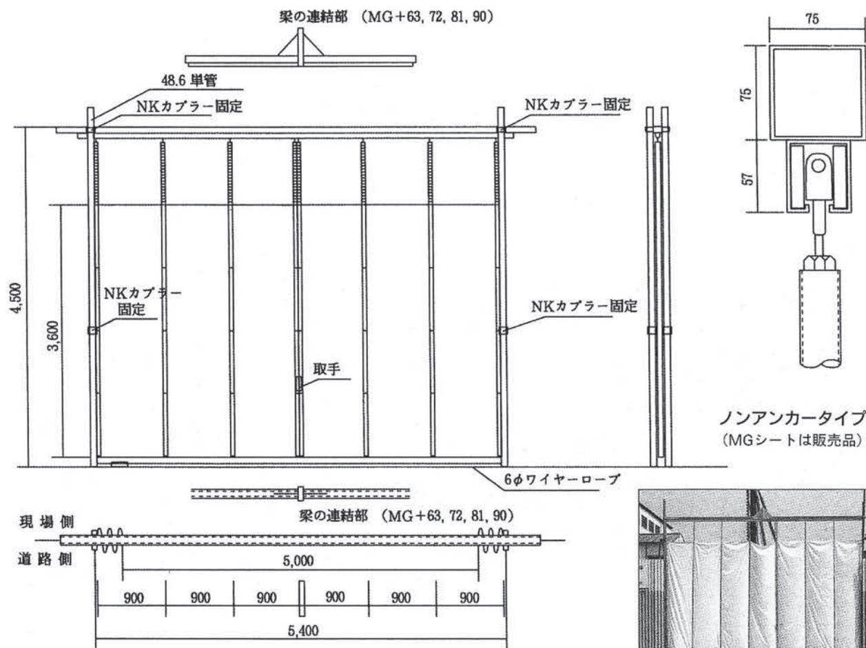
■シートゲート部材表
