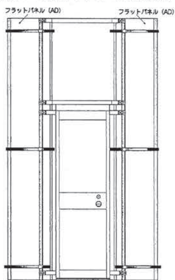
●ドアパネルとフラットパネルの取付図
