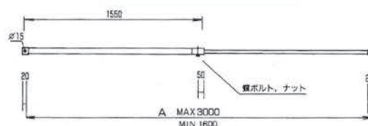
鉄骨階段伸縮手摺D型
