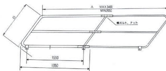
鉄骨階段手摺1型
