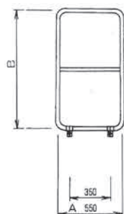
鉄骨階段手摺3型
