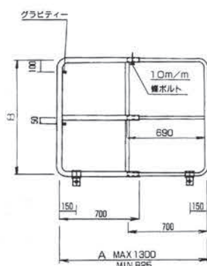
鉄骨階段手摺2型
