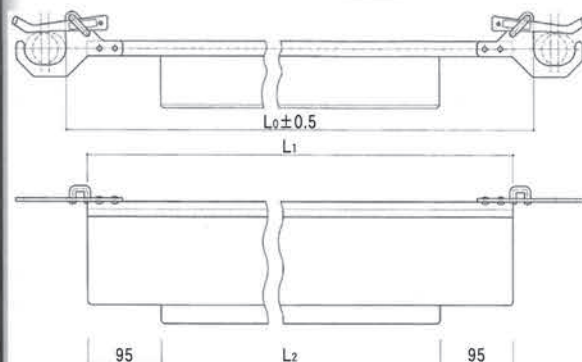
建枠足場(φ42.7mm)用
