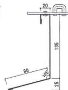
建枠足場(φ42.7mm)用
